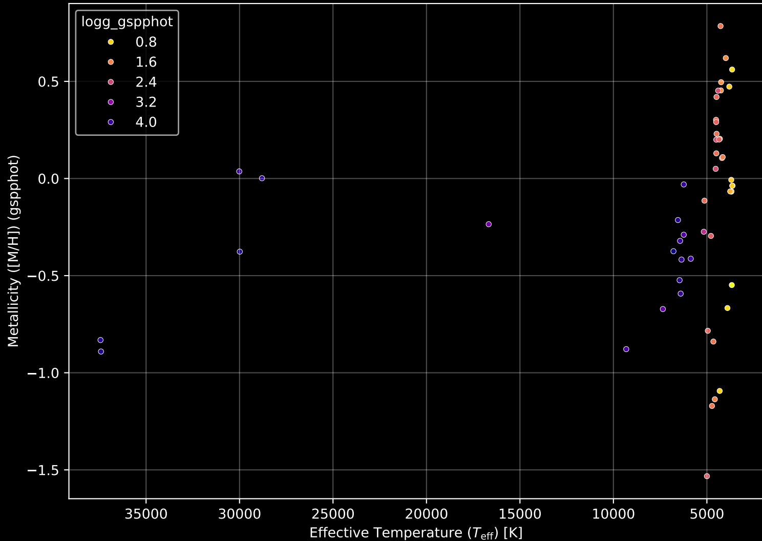
APOGEE DR17 Field: [283-34-O] Stellar Population Parameters (n= 52)
