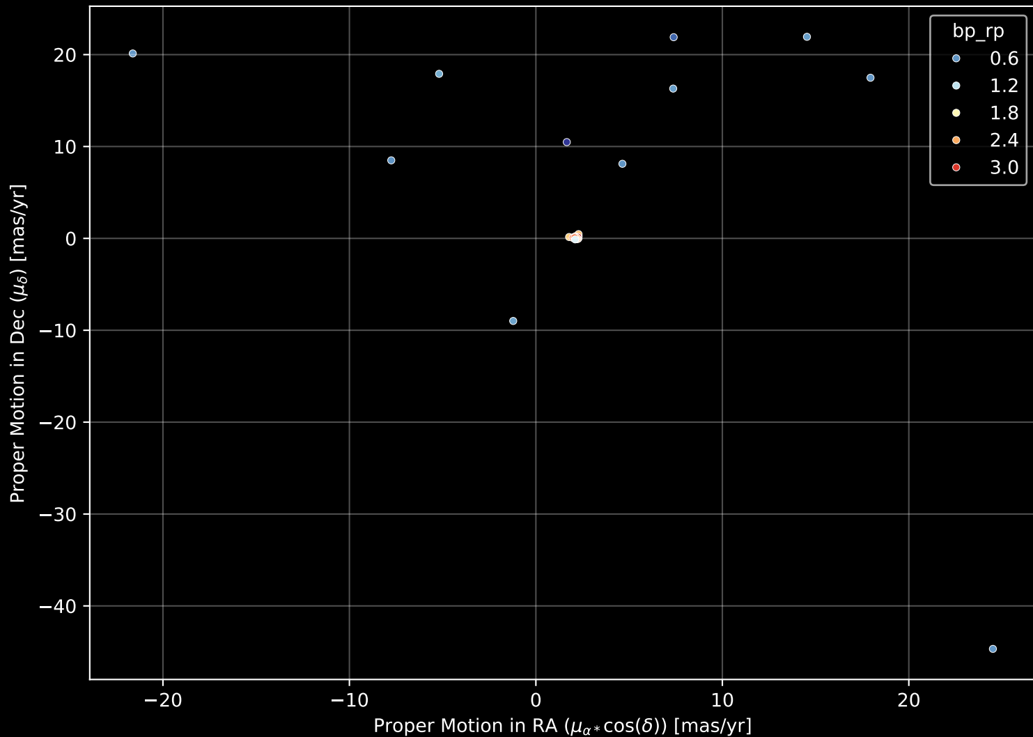
APOGEE DR17 Field: [283-34-O] Proper Motion Diagram (n= 52)
