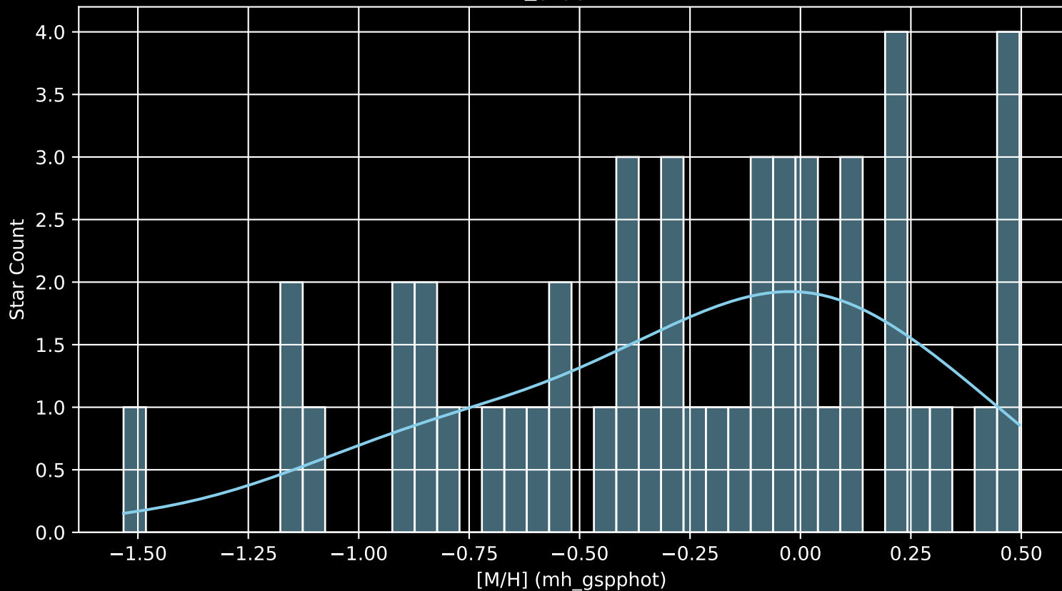
APOGEE DR17 Field: [283-34-O [M/H] (mh_gspphot) (n= 49)
